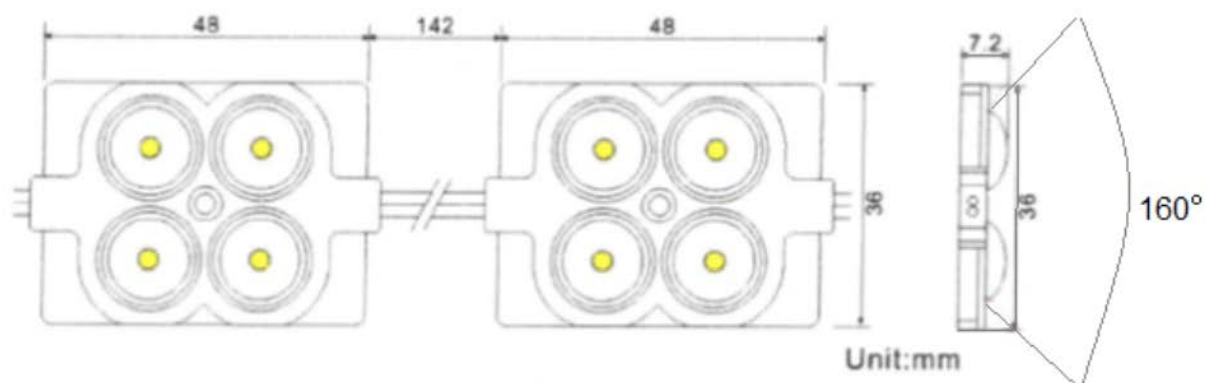
Figur 2-2: LED modul, mål i mm
