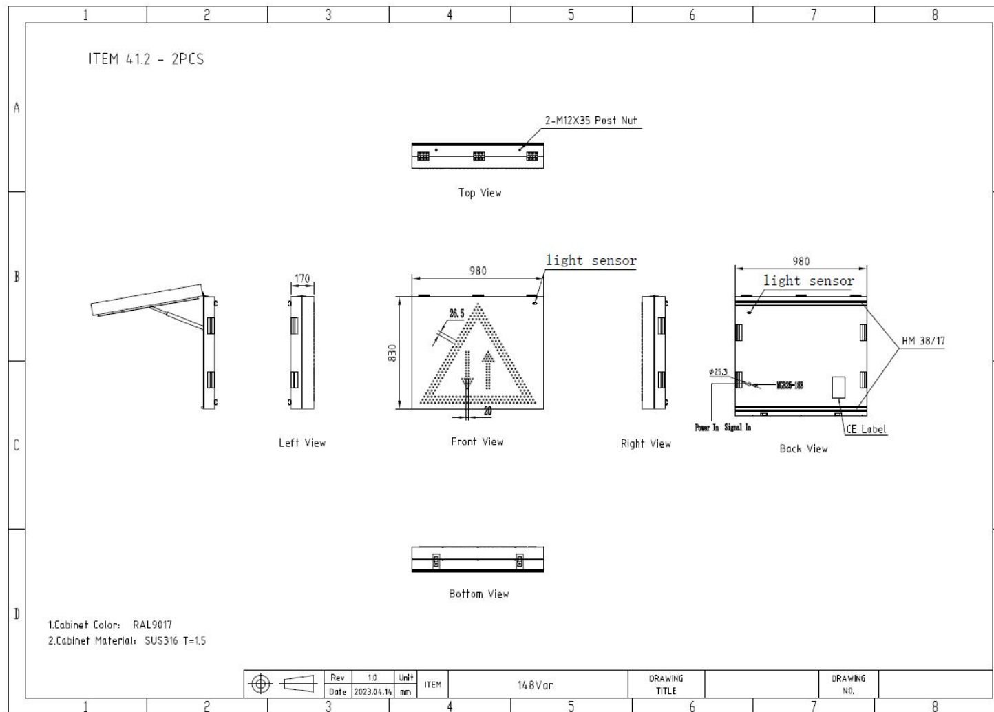
Figur 1: Sammenstillingstegning (GA)
